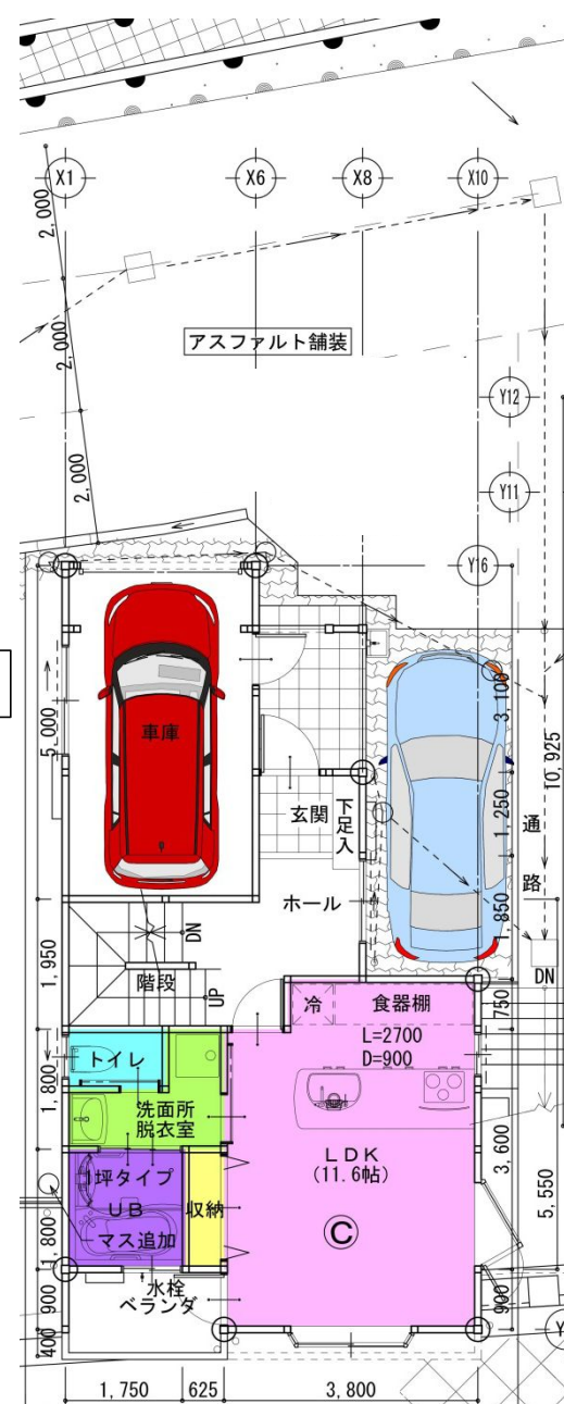
1階平面図
